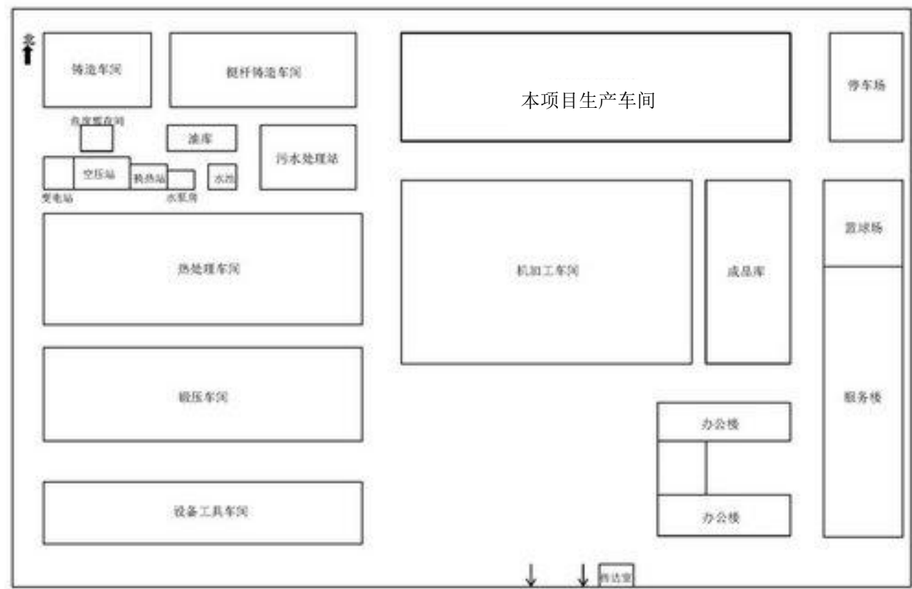
附图 2 项目厂区平面布置图
